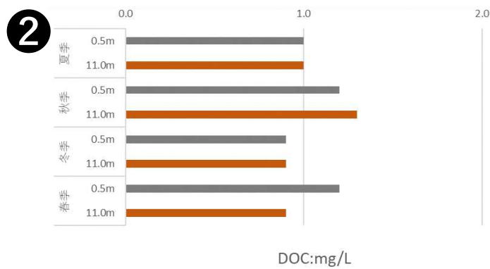
図Ⅱ-1-(4)-6 各地点・四季の有機物及び栄養塩類等の濃度 (DOC)
