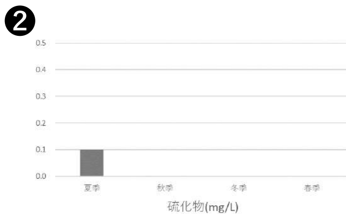
図Ⅱ-1-(4)-8 各地点・四季の底質溶出量の分析結果（硫化物）
