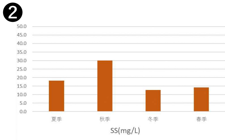
図Ⅱ-1-(4)-8 各地点・四季の底質溶出量の分析結果 (SS)
