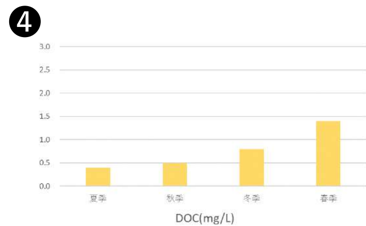
図Ⅱ-1-(4)-8 各地点・四季の底質溶出量の分析結果 (DOC)
