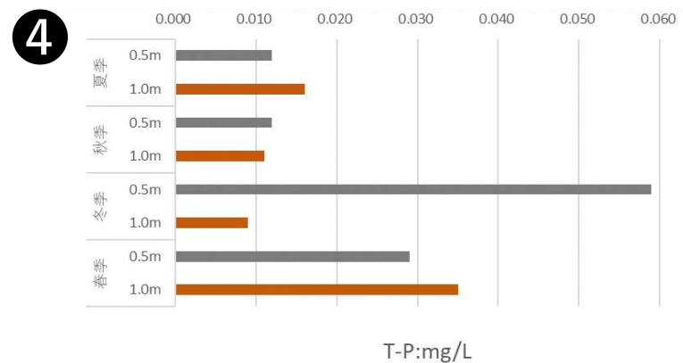
図Ⅱ-1-(4)-6 各地点・四季の有機物及び栄養塩類等の濃度 (T-P)
