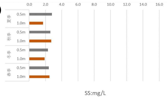
図Ⅱ-1-(4)-6 各地点・四季の有機物及び栄養塩類等の濃度 (SS)
