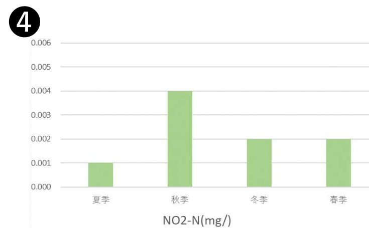
図Ⅱ-1-(4)-8 各地点・四季の底質溶出量の分析結果 (NO 2 -N)
