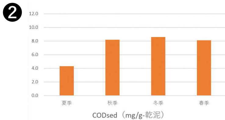
図Ⅱ-1-(4)-7 各地点・四季の底質含有量の量 (COD)
