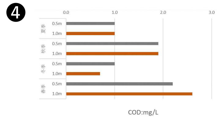
図Ⅱ-1-(4)-6 各地点・四季の有機物及び栄養塩類等の濃度 (COD)
