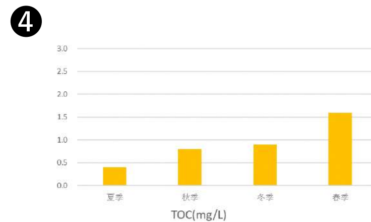
図Ⅱ-1-(4)-8 各地点・四季の底質溶出量の分析結果 (TOC)
