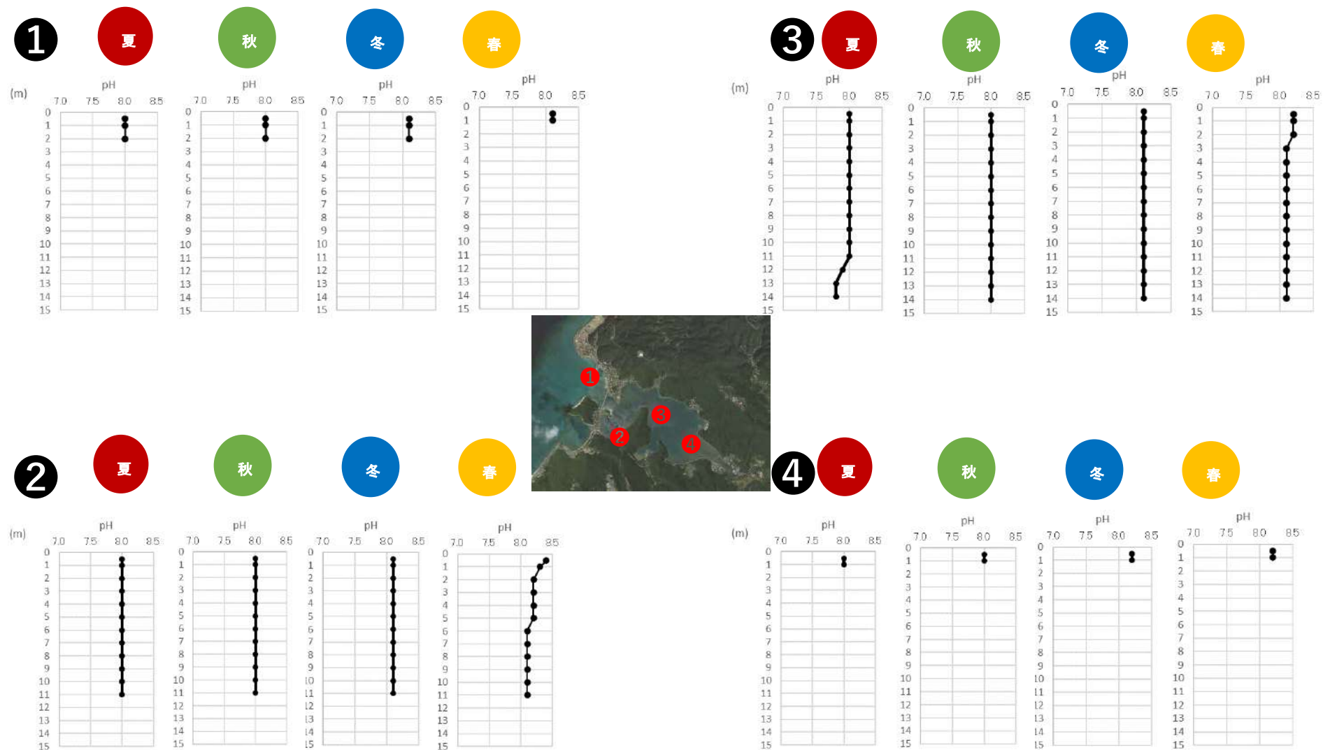
図Ⅱ-1-(4)-4 各地点・四季の pH 鉛直分布図
