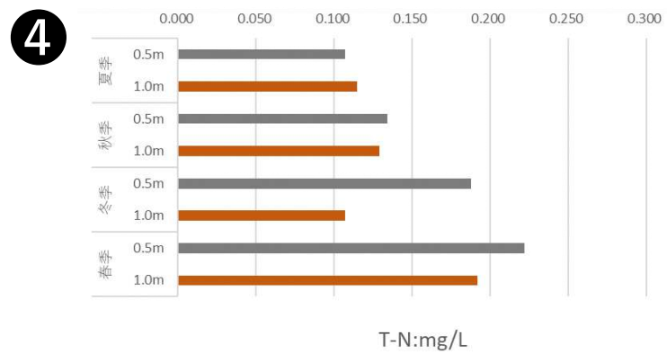
図Ⅱ-1-(4)-6 各地点・四季の有機物及び栄養塩類等の濃度 (T-N)
