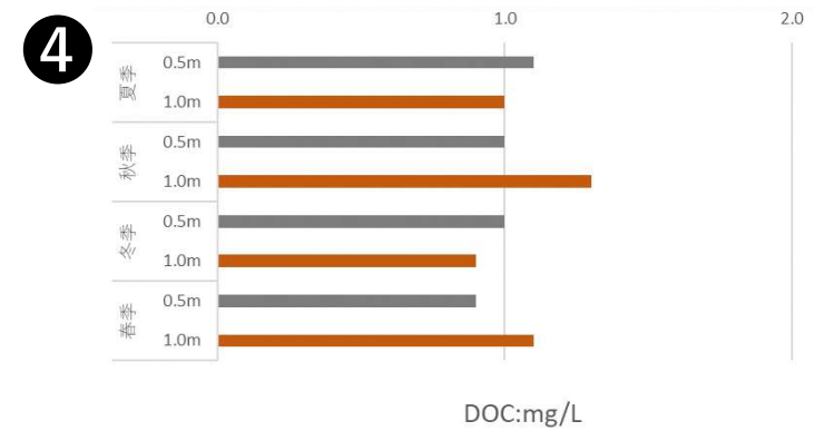
図Ⅱ-1-(4)-6 各地点・四季の有機物及び栄養塩類等の濃度 (DOC)
