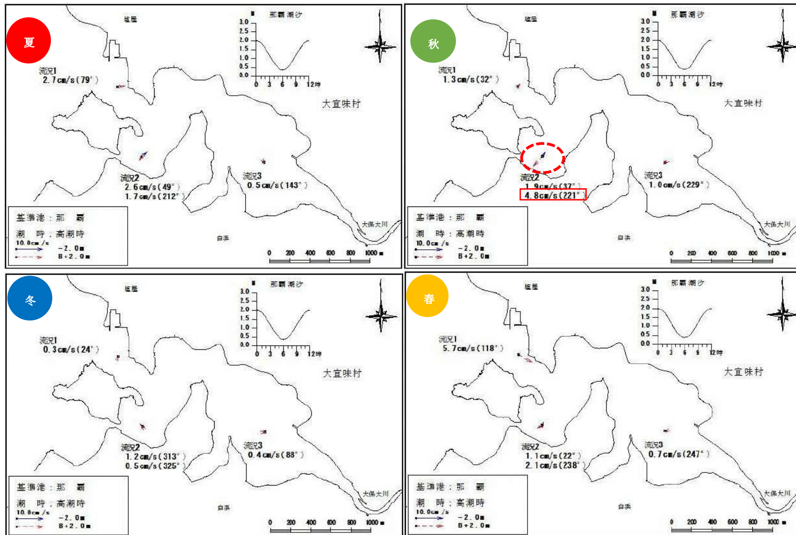
図Ⅱ-1-(3)-5 平均大潮期流況 (満潮時)
