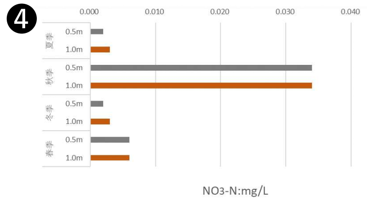
図Ⅱ-1-(4)-6 各地点・四季の有機物及び栄養塩類等の濃度 (NO 3 -N)
