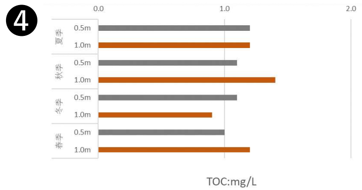
図Ⅱ-1-(4)-6 各地点・四季の有機物及び栄養塩類等の濃度 (TOC)
