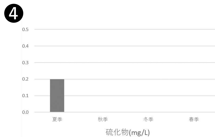
図Ⅱ-1-(4)-8 各地点・四季の底質溶出量の分析結果（硫化物）
