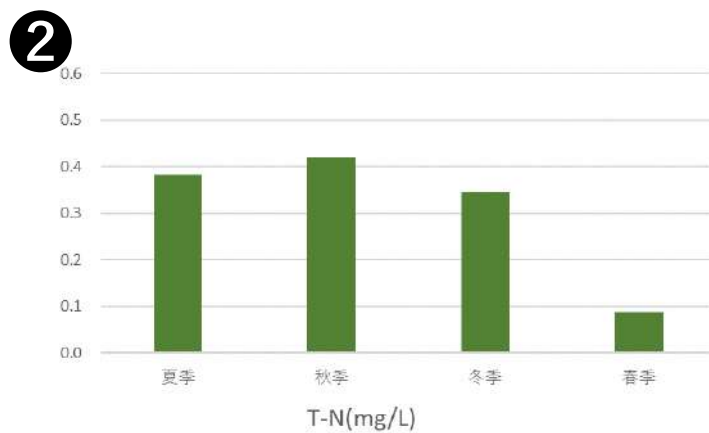
図Ⅱ-1-(4)-8 各地点・四季の底質溶出量の分析結果 (T-N)
