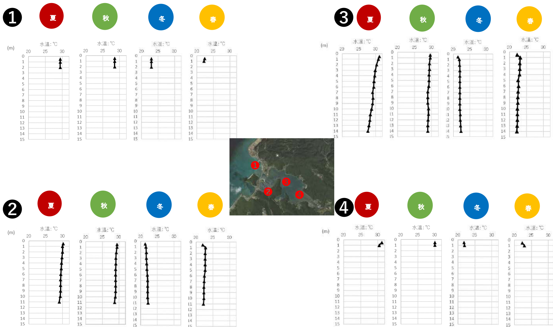
図Ⅱ-1-(4)-2 各地点・四季の水溫鉛直分布図
