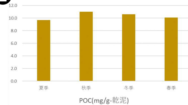
図Ⅱ-1-(4)-8 各地点・四季の底質含有量の量 (POC)
