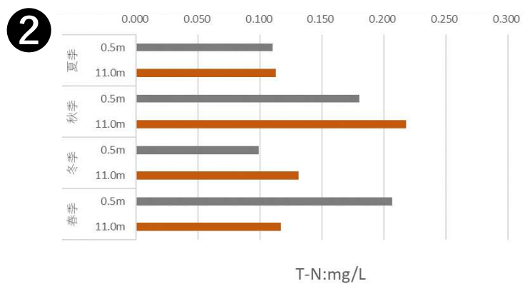
図Ⅱ-1-(4)-6 各地点・四季の有機物及び栄養塩類等の濃度 (T-N)
