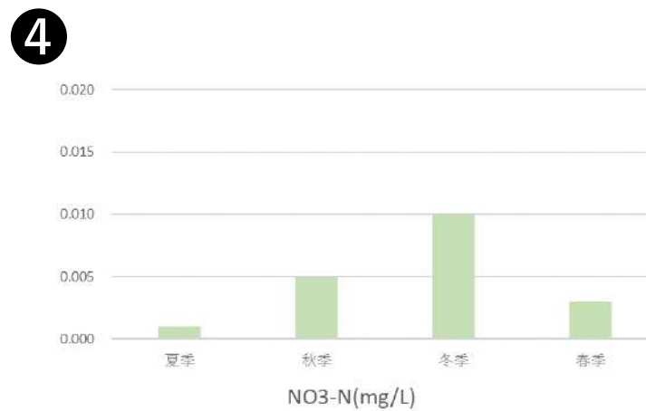
図Ⅱ-1-(4)-8 各地点・四季の底質溶出量の分析結果 (NO 3 -N)
