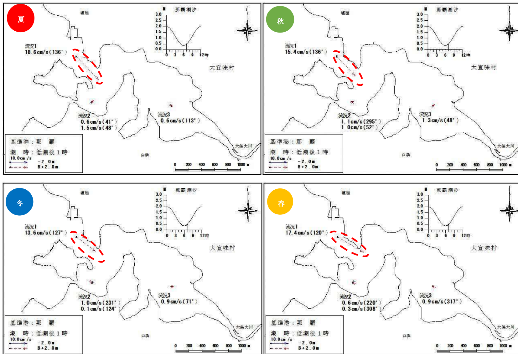
図 II-1-(3)-8 平均大潮期流況 (上げ潮となった 1 時間後)
