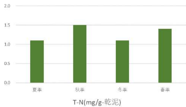
図Ⅱ-1-(4)-8 各地点・四季の底質含有量の量 (T-N)
