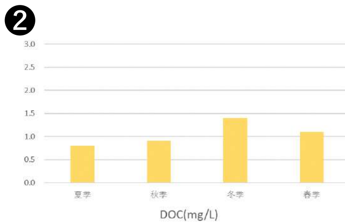
図Ⅱ-1-(4)-8 各地点・四季の底質溶出量の分析結果 (DOC)
