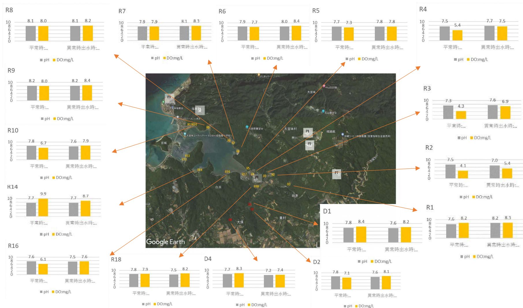
図Ⅱ-2- (2) -6 その他流入河川の水質（平水時及び異常出水時）
