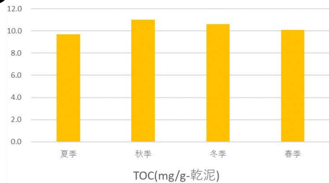
図Ⅱ-1-(4)-8 各地点・四季の底質含有量の量 (TOC)
