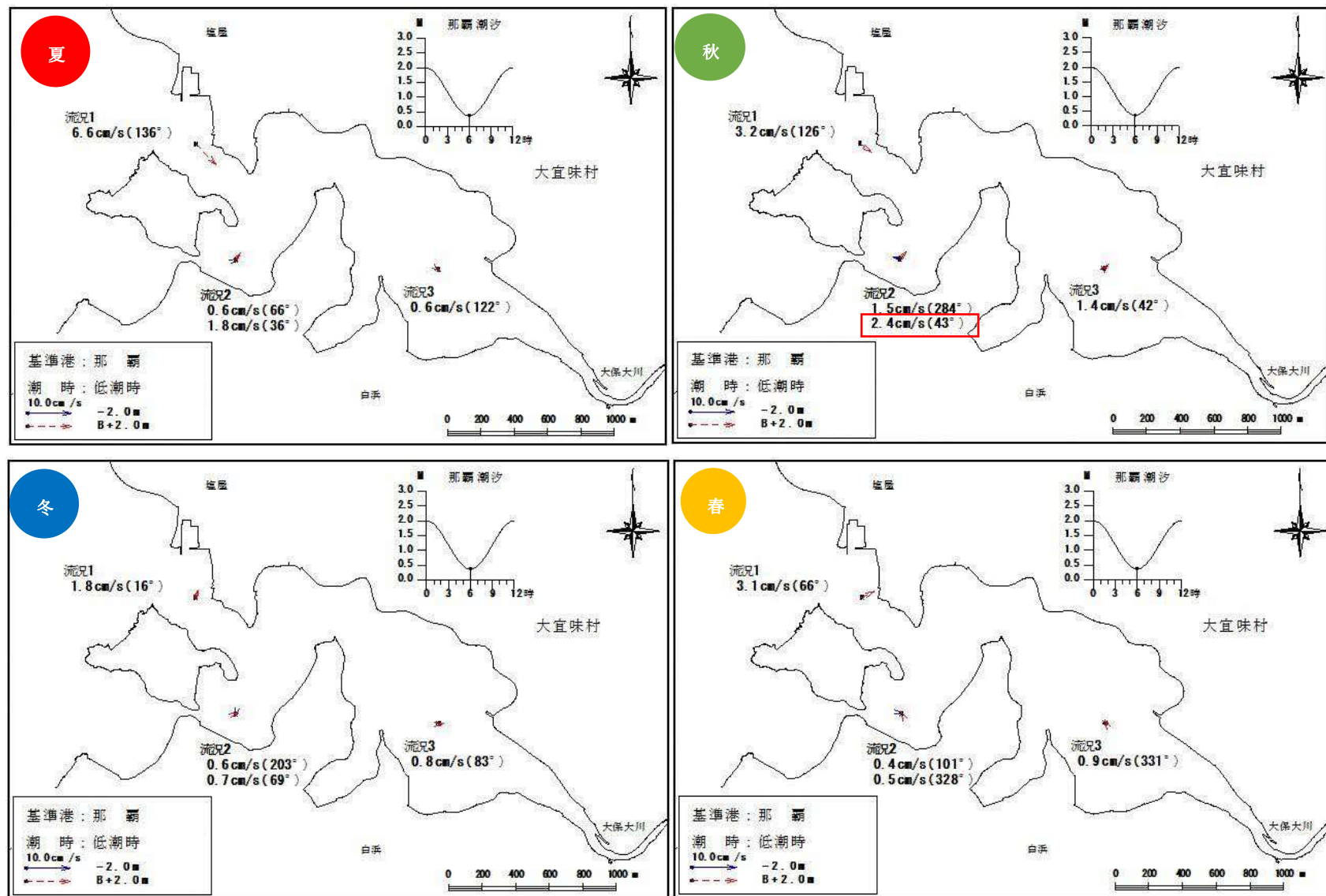
図Ⅱ-1-(3)-7 平均大潮期流況（干潮時）
