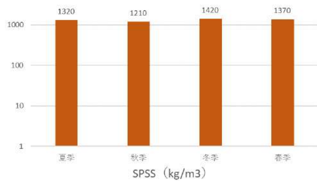
図Ⅱ-1-(4)-7 各地点・四季の底質含有量の量 (SPSS)
