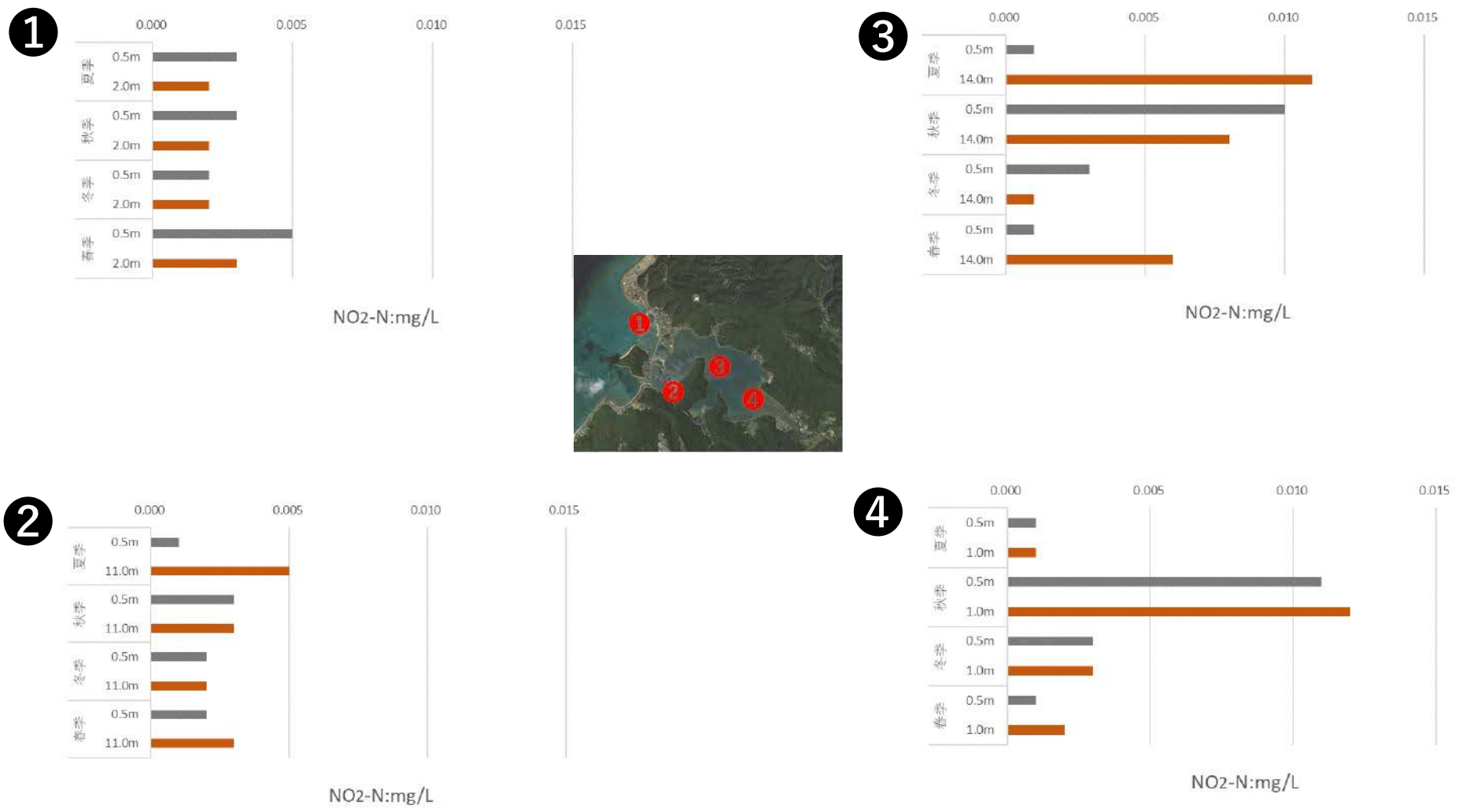
図Ⅱ-1-(4)-6 各地点・四季の有機物及び栄養塩類等の濃度 (NO 2 -N)
