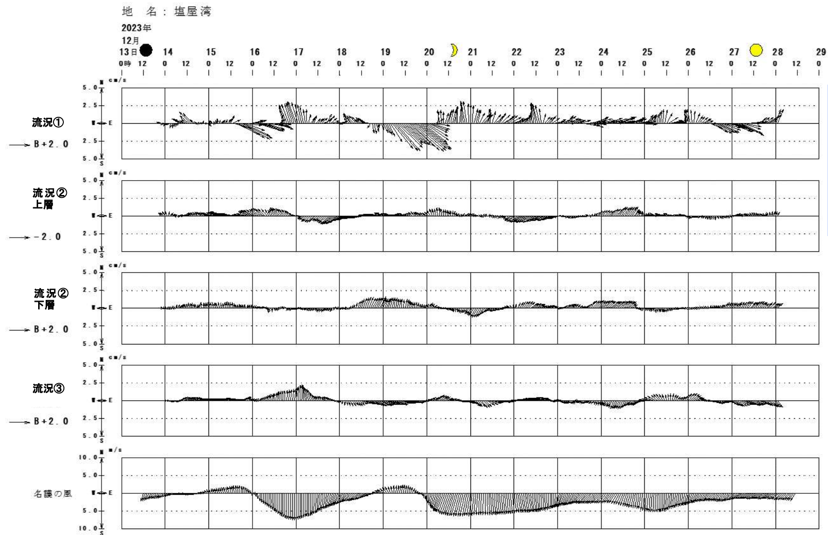
図Ⅱ-1-(3)-4 各地点（層）における25時間移動平均ベクトル図（時間毎の流向流速及び名護の風）-3：冬季
