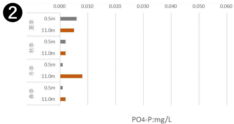
図Ⅱ-1-(4)-6 各地点・四季の有機物及び栄養塩類等の濃度 (PO 4 -P)
