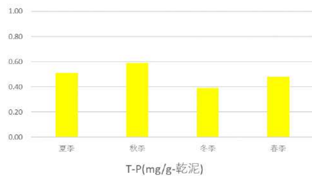
図Ⅱ-1-(4)-8 各地点・四季の底質含有量の量 (T-P)
