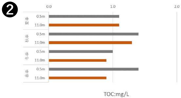
図Ⅱ-1-(4)-6 各地点・四季の有機物及び栄養塩類等の濃度 (TOC)
