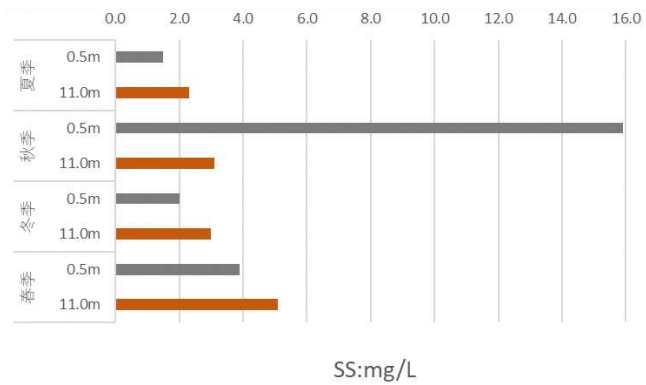
図Ⅱ-1-(4)-6 各地点・四季の有機物及び栄養塩類等の濃度 (SS)
