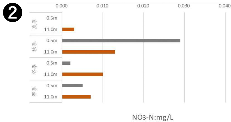
図Ⅱ-1-(4)-6 各地点・四季の有機物及び栄養塩類等の濃度 (NO 3 -N)
