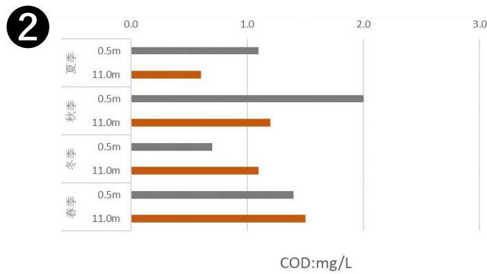
図Ⅱ-1-(4)-6 各地点・四季の有機物及び栄養塩類等の濃度 (COD)
