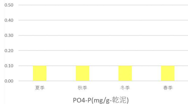
図Ⅱ-1-(4)-8 各地点・四季の底質含有量の量 (PO 4 -P)
