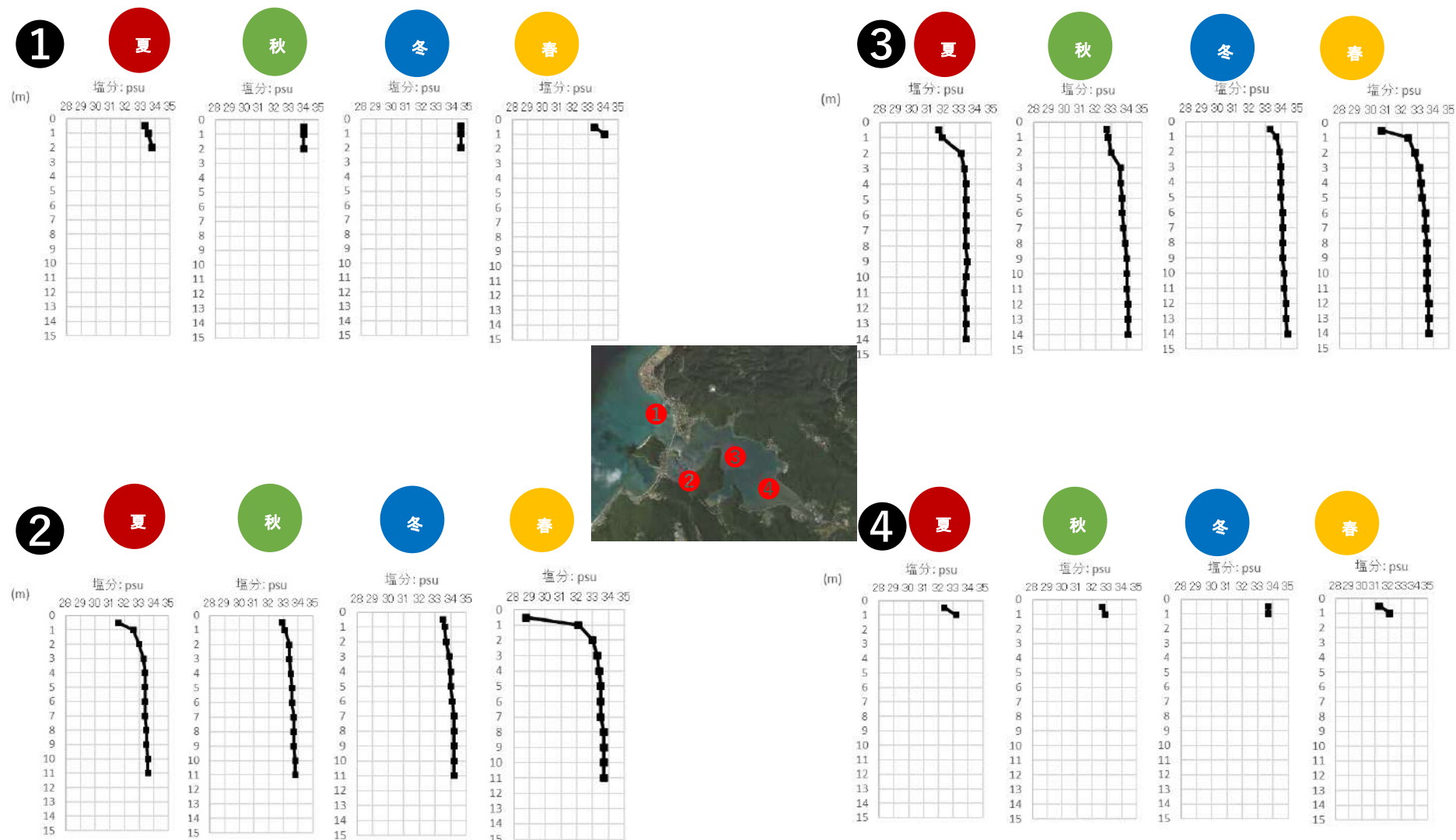
図Ⅱ-1-(4)-3 各地点・四季の塩分鉛直分布図
