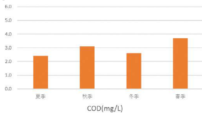
図Ⅱ-1-(4)-8 各地点・四季の底質溶出量の分析結果 (COD)
