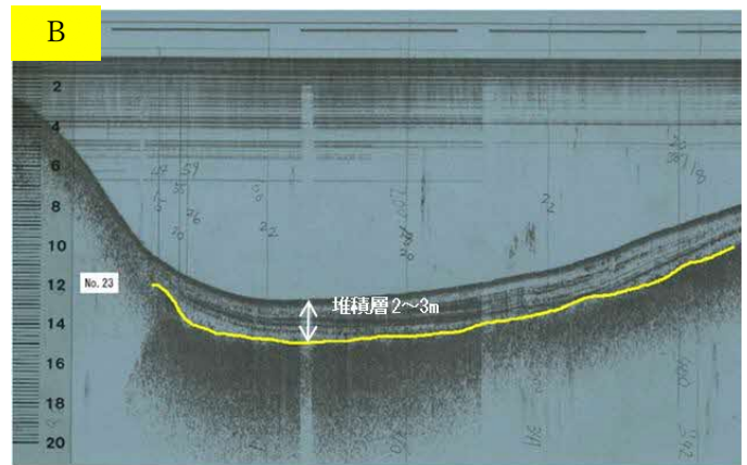
図Ⅱ-1-(2)-6 シルト分の堆積層（断面図）
