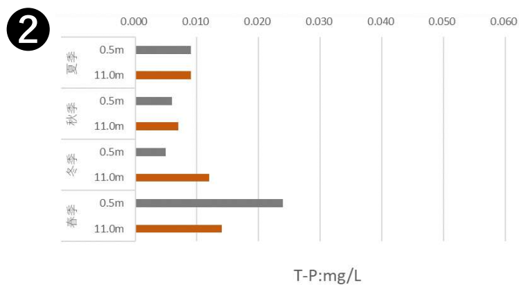
図Ⅱ-1-(4)-6 各地点・四季の有機物及び栄養塩類等の濃度 (T-P)
