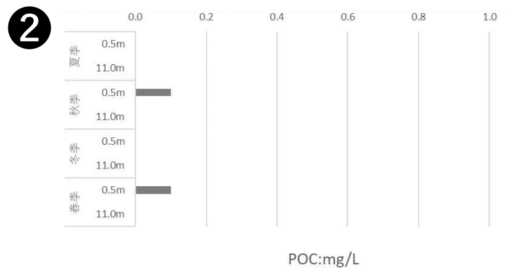
図Ⅱ-1-(4)-6 各地点・四季の有機物及び栄養塩類等の濃度 (POC)
