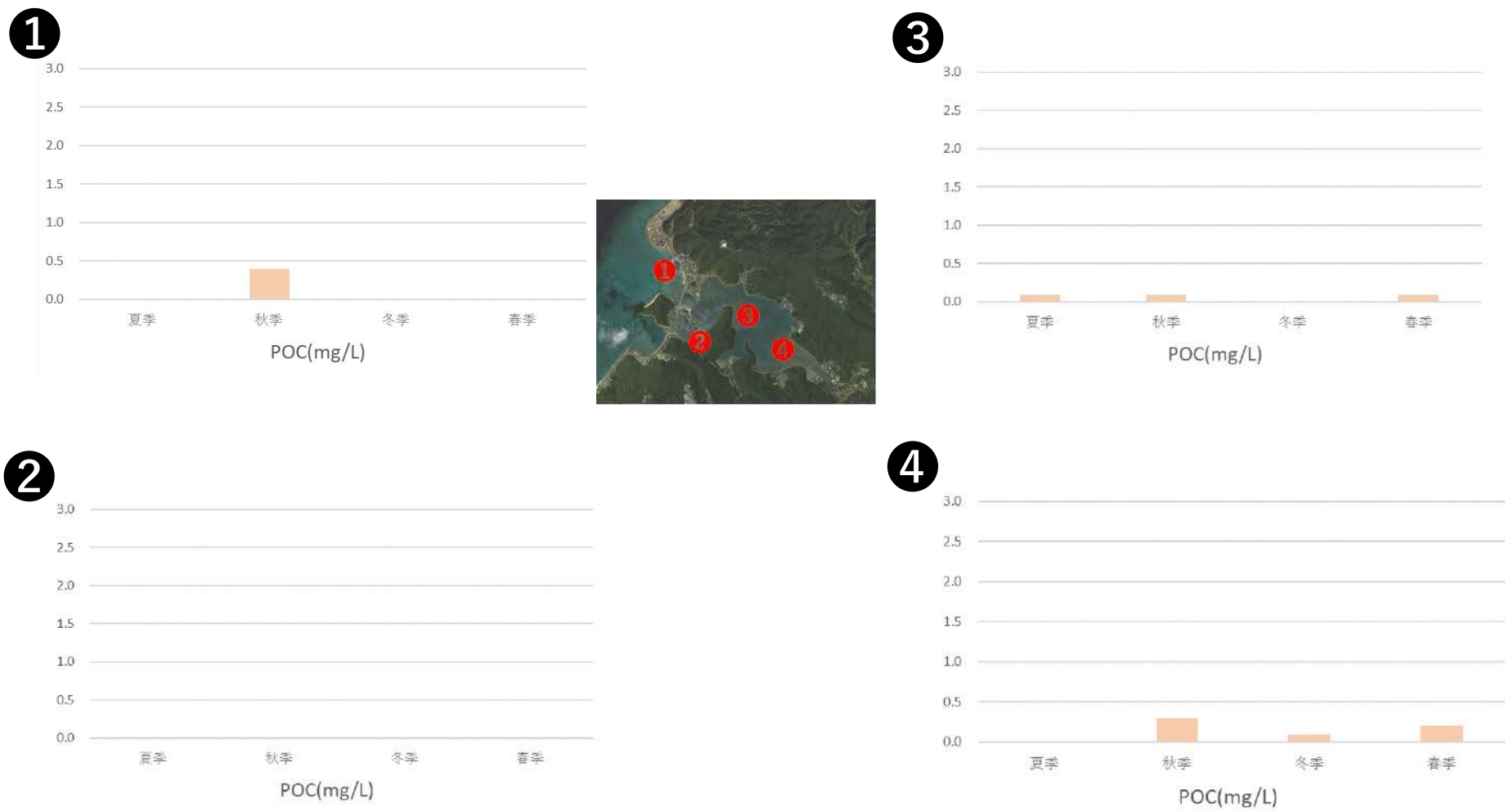
図Ⅱ-1-(4)-8 各地点・四季の底質溶出量の分析結果 (POC)
